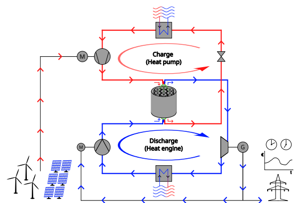
Aufbau und Einbindung einer Carnot-Batterie
