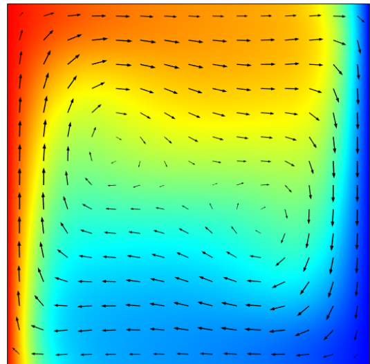
Beispiel: Natürliche Konvektion in einem Viereckbehälter
